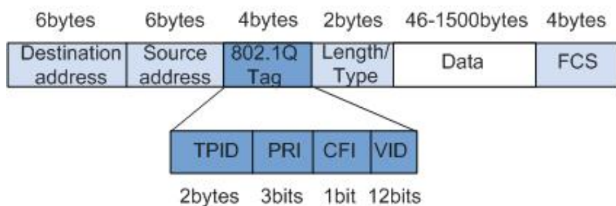
802.1Q Tag 各字段含义介绍
