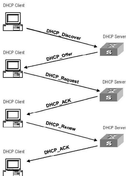
图 1-2. DHCP Client 与 DHCP Server 间的报文交互过程
